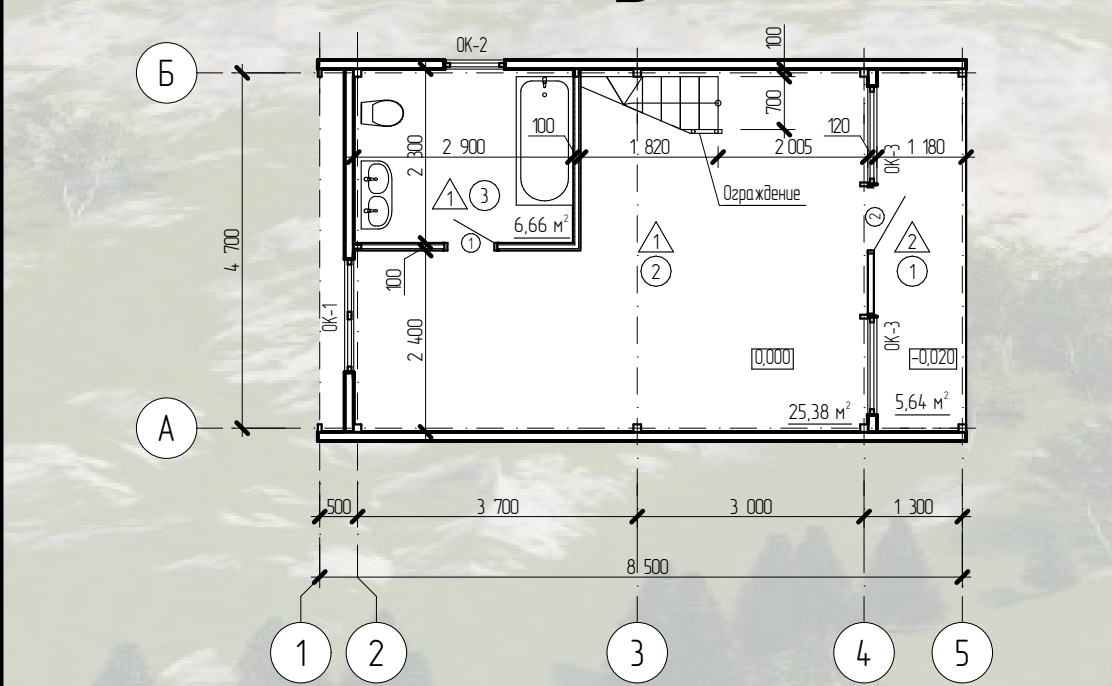
План антресоли гостевого дома №2
