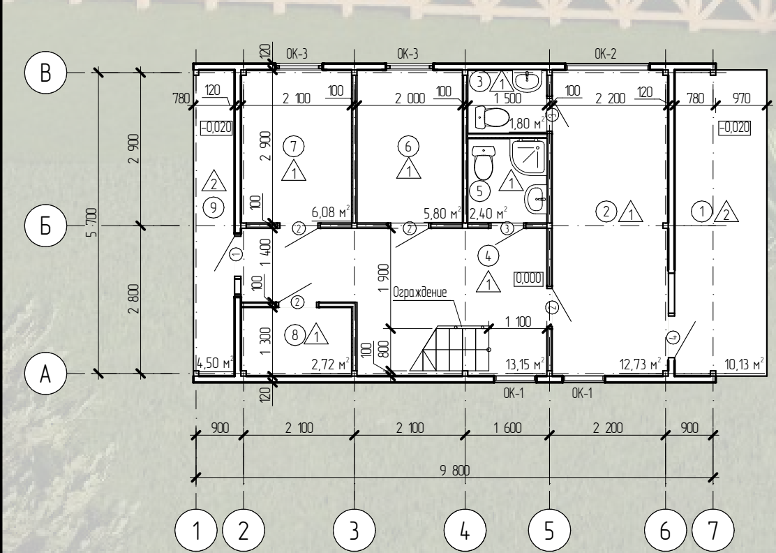
План второго этажа администрации
