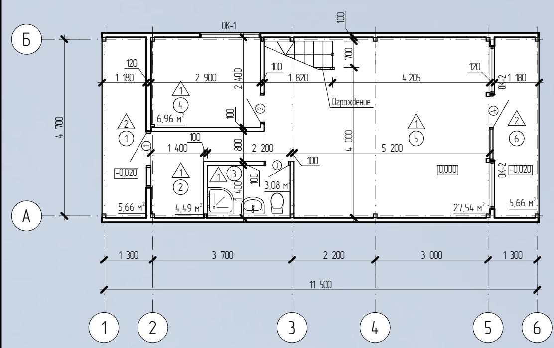
План антресоли гостевого дома №1
