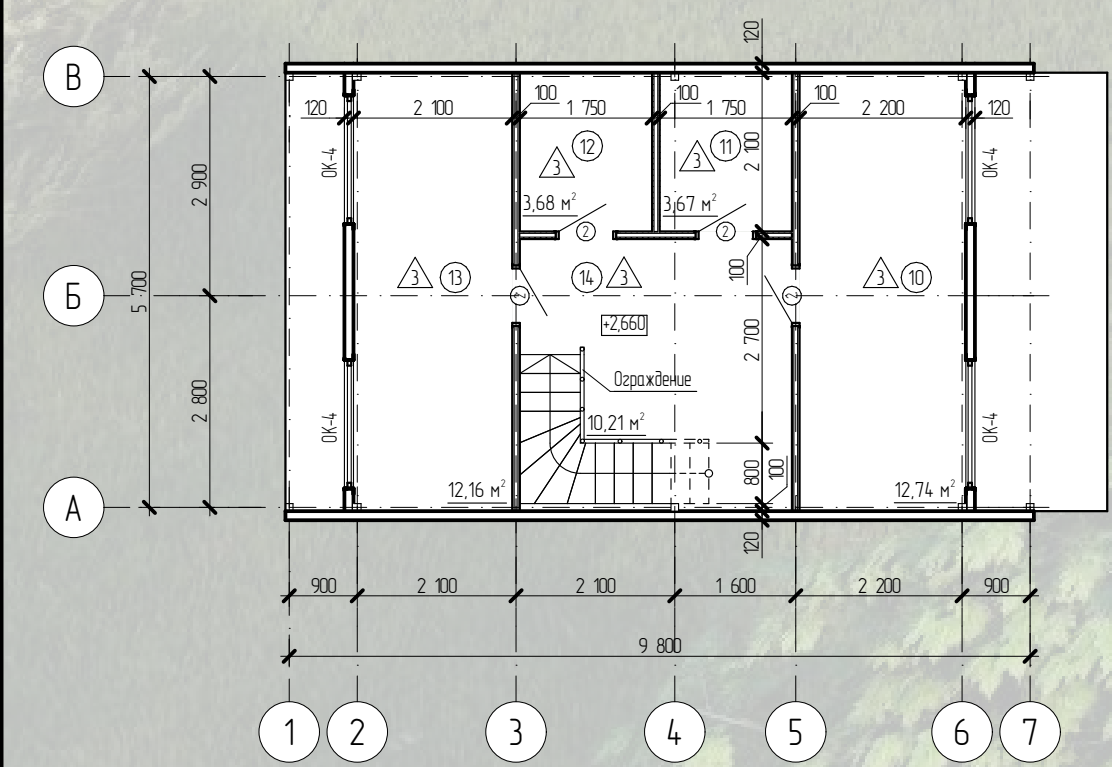
План второго этажа администрации
