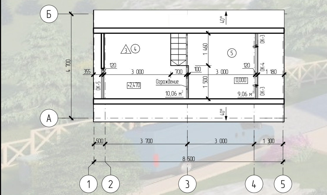
План первого этажа администрации
